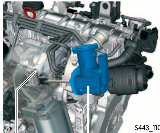
Ladedrucksteller V465
