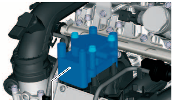
Zündtrafo N152
