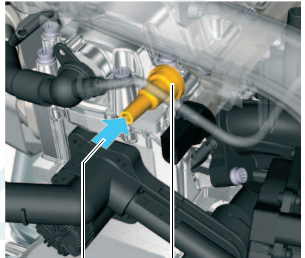
Luftzuführung vom Luftfilter Rückschlagventil S443_108
