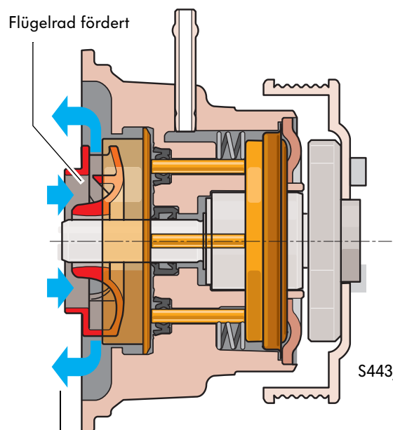
Kühlmittel-Förderstrom zum Zylinderblock und Zylinderkopf
