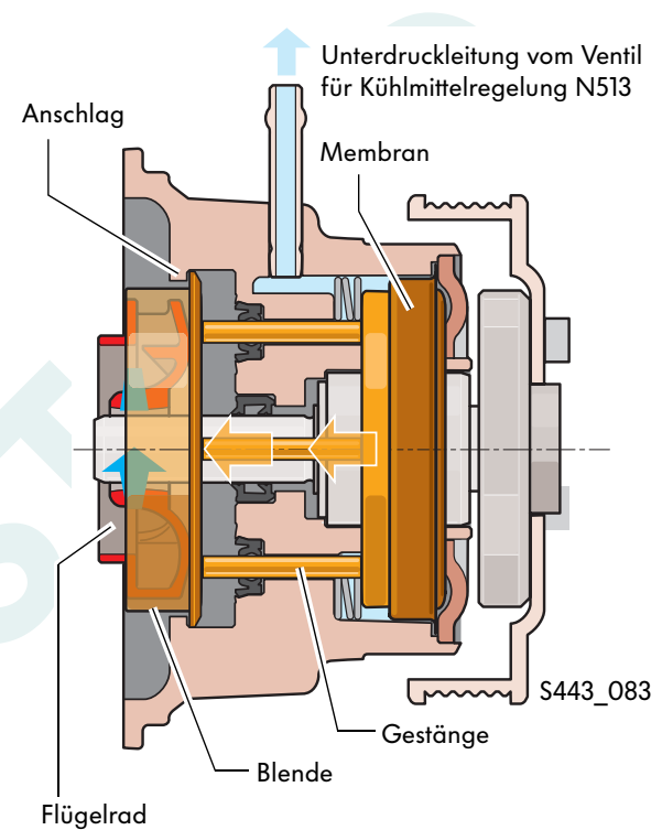
Der Kühlmittel-Förderstrom wird durch die Blende abgeblockt.
