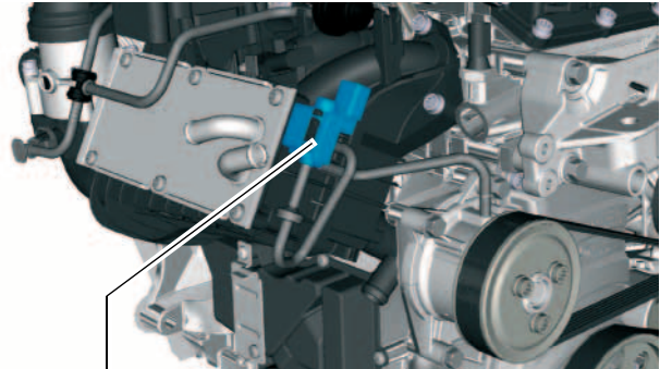
Ventil für Kühlmittelregelung N513
