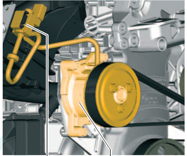
Ventil für Kühlmittelregelung N513
